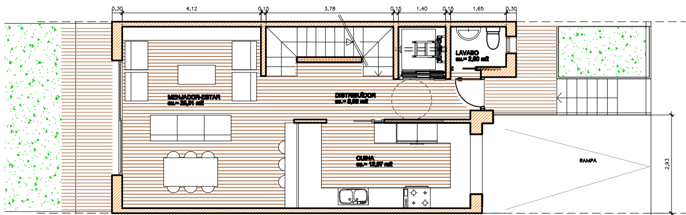
PLANTA BAIXA
